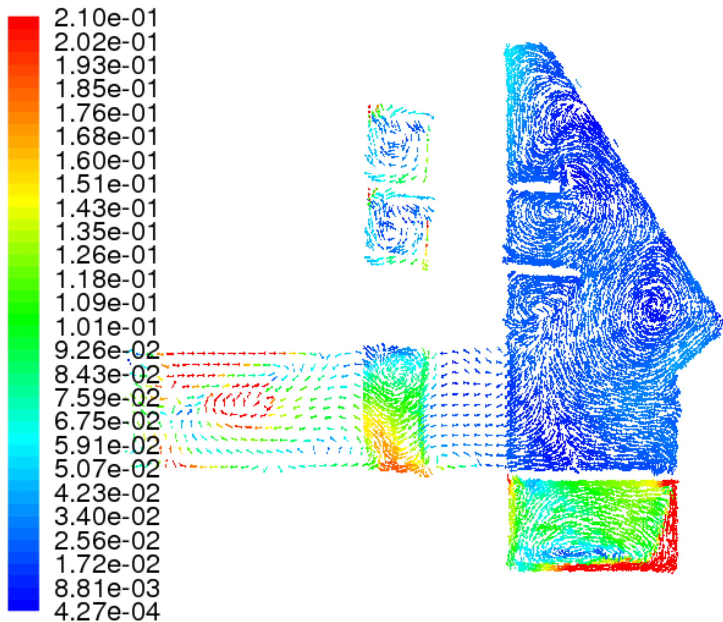
Vectores de velocidad (m/s) en un plano vertical que corta a las salas de espera de planta baja
