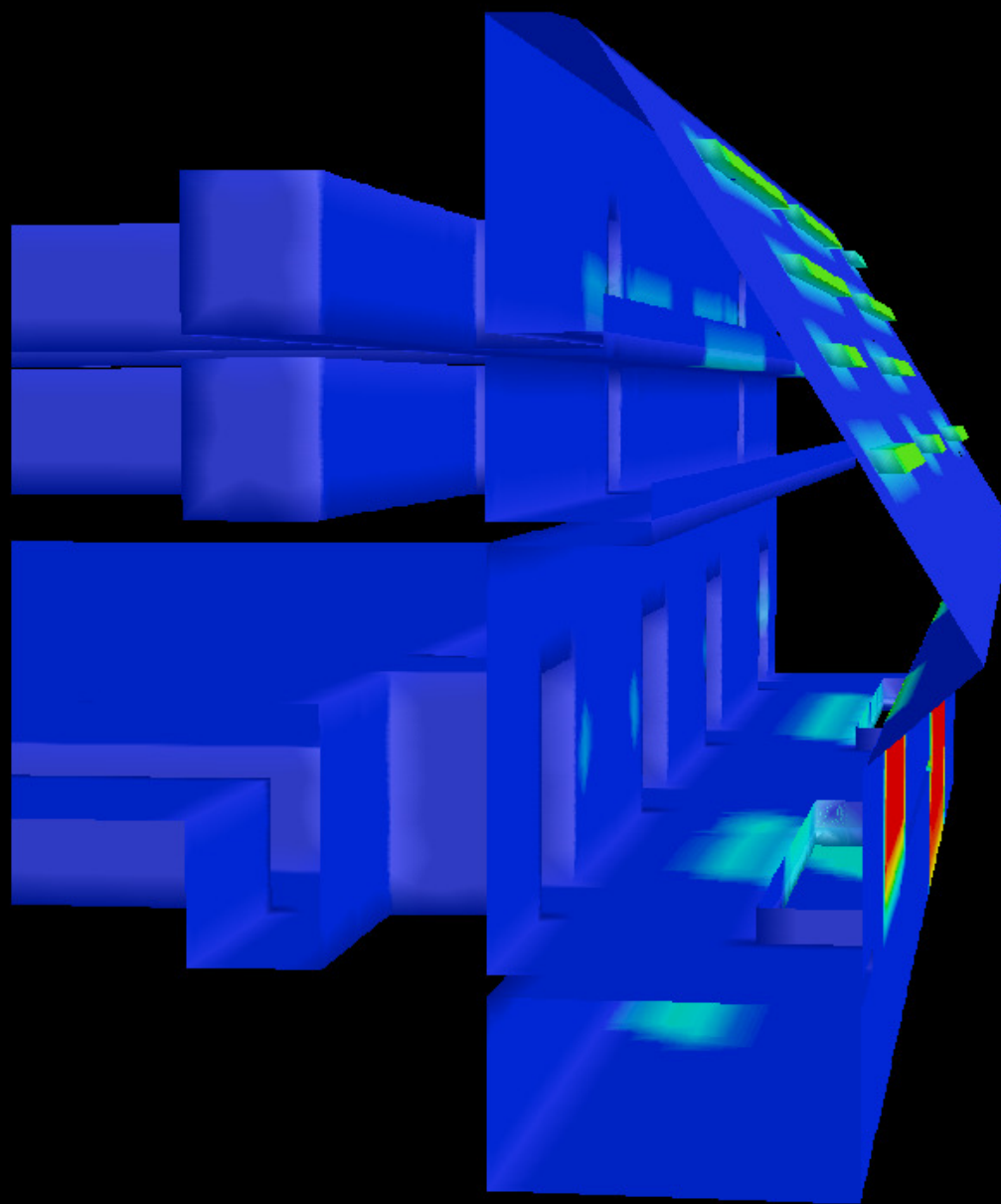
Flujo de calor por radiación solar directa en el interior del recinto ( W/m^2 )
